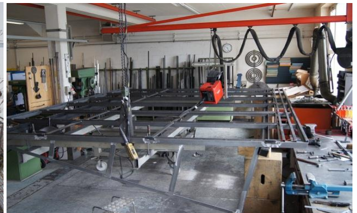
Die Dachkonstruktion wird in der Werkstatt zusammen geschweisst.
